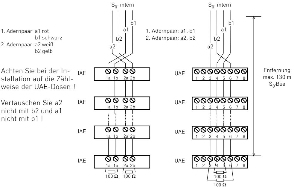
Verdrahtung eines internen S 0 -Anschlusses
