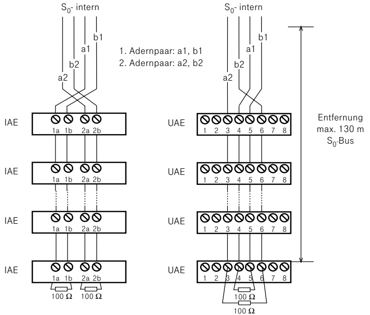
Verdrahtung eines internen S 0 -Anschlusses
