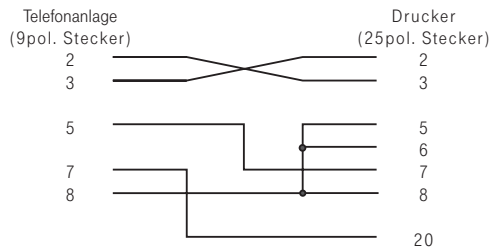
Abb. 7: Anschlussbelegung - Drucker-kabel
